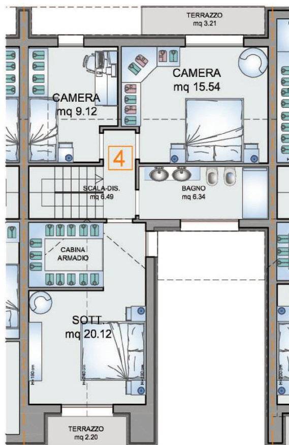
PIANO PRIMO/SOTTOTETTO
