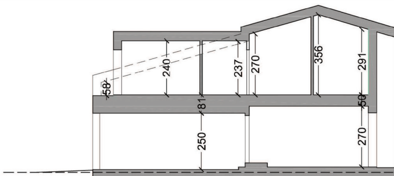
SEZIONE TIPO
